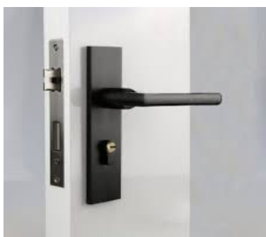
Serrure mortaisée dans l'épaisseur de la porte
